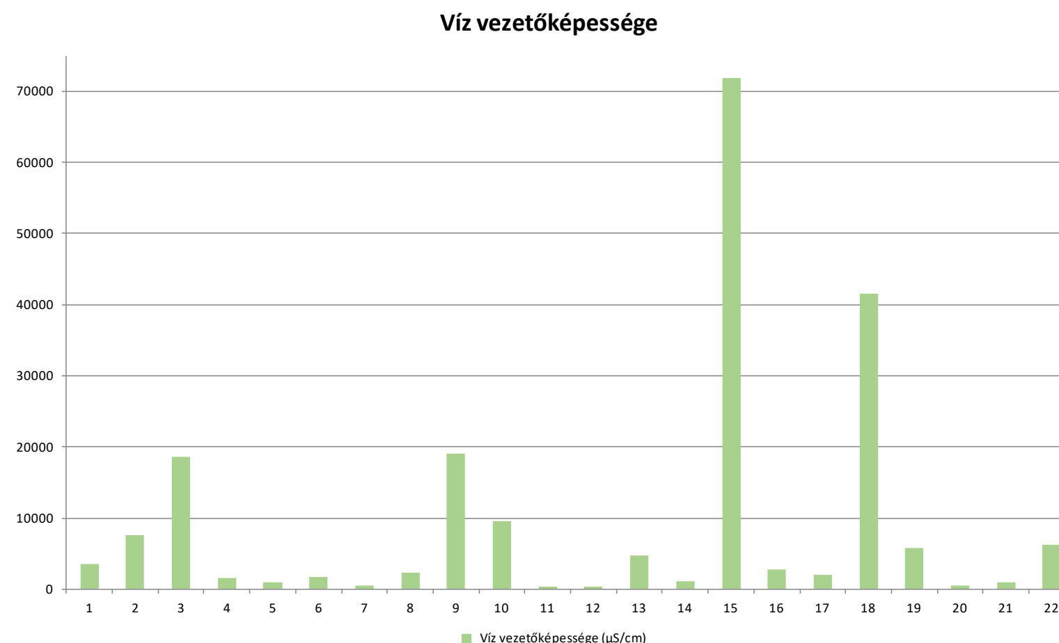
16. ábra. A tavak vizének vezetőképessége ( \mu\text{S}/\text{cm} ) / Figure 16. Conductivity of water of lakes ( \mu\text{S}/\text{cm} )
